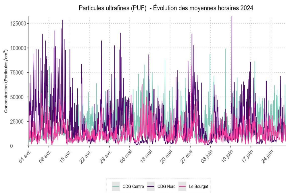
Figure 6: Particules ultrafines sur Paris-Charles de Gaulle et Paris-Le Bourget - Evolution des moyennes horaires
