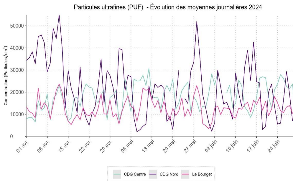
Figure 7: Particules ultrafines sur Paris-Charles de Gaulle et Paris-Le Bourget - Evolution des moyennes journalières
