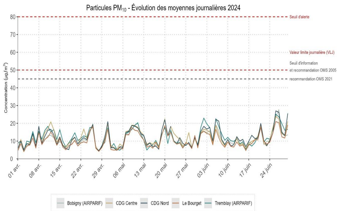
Figure 4: PM10 sur Paris-Charles de Gaulle, Paris-Le Bourget et environs - Evolution des moyennes journalières
