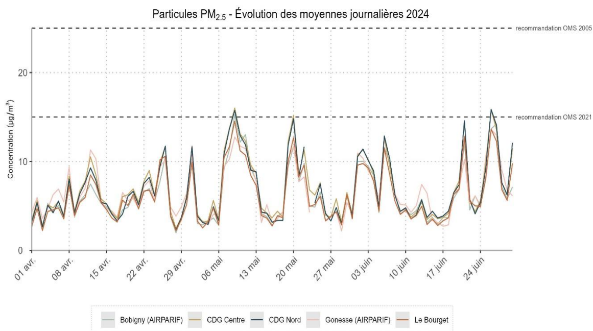
Figure 5: PM 2,5 sur Paris-Charles de Gaulle, Paris-Le Bourget et environs - Evolution des moyennes journalières
