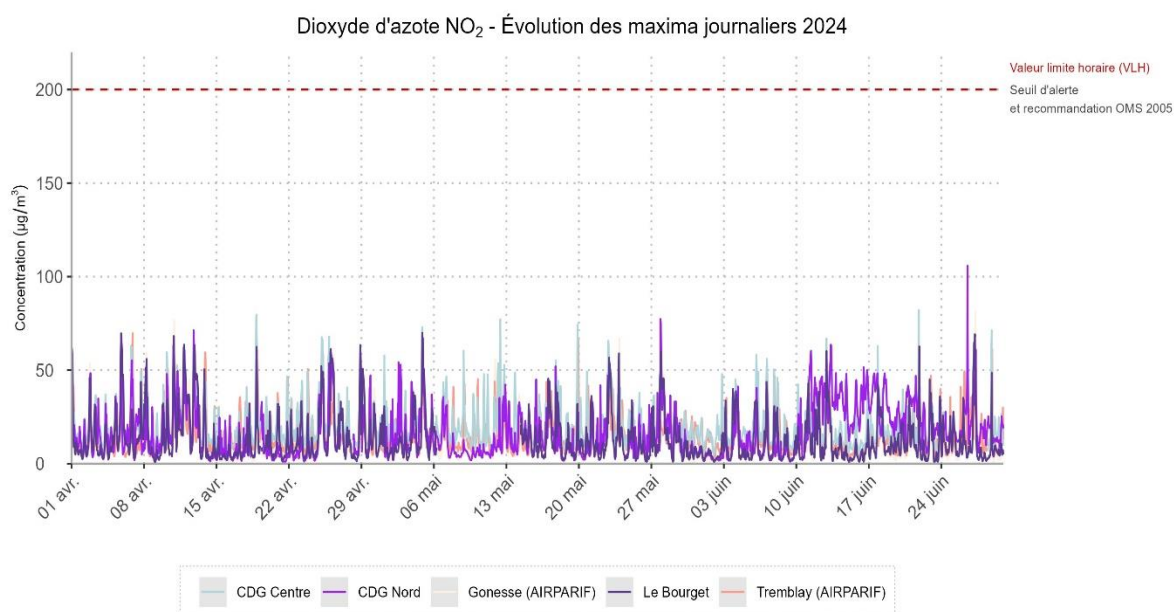
Figure 2: Dioxyde d'azote (NO 2 ) sur Paris-Charles de Gaulle, Paris-Le Bourget et environs - Evolution des maxima horaires journaliers
