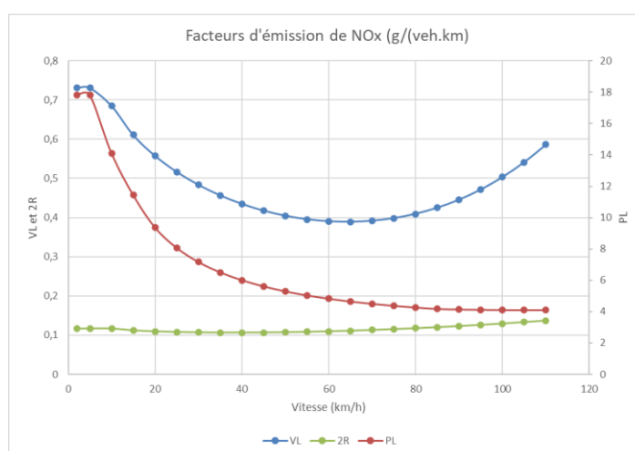
Figure 20: Facteurs d'émission en fonction de la vitesse pour les NOx sur la base des facteurs COPERT V et du parc UGE-IFSTAR-2020.
