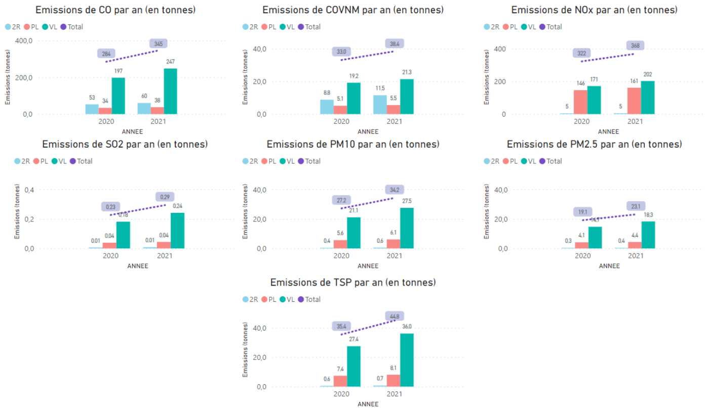
Figure 21: Emissions totales sur les années 2020 et 2021 issues du trafic routier en zone publique, par polluant et par catégorie de véhicule (2R, VL, PL) ainsi que le total des émissions sur la plateforme Paris-Charles de Gaulle
