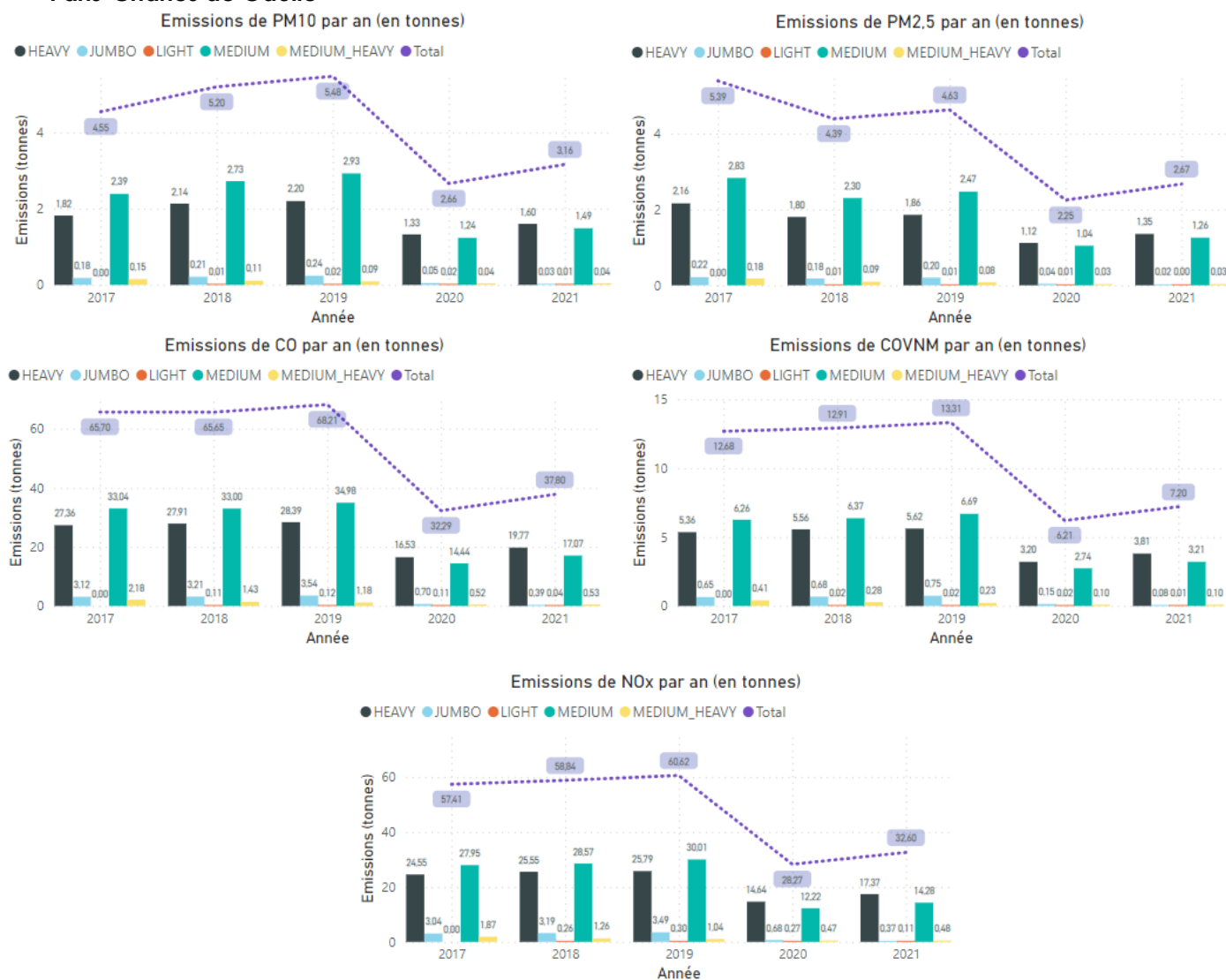
Figure 14 : Evolution pluriannuelle des émissions en tonnes de CO, NOx, COVNM et PM10 / PM2.5 avec les facteurs CDG 2018 pour la plateforme de Paris-Charles de Gaulle
