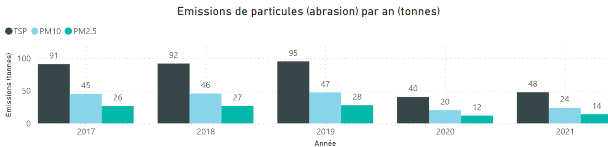
Figure 6 : Evolution annuelle des émissions de polluants issues de l'abrasion (TSP, PM 10 , PM 2,5 ) à Paris-Charles de Gaulle
