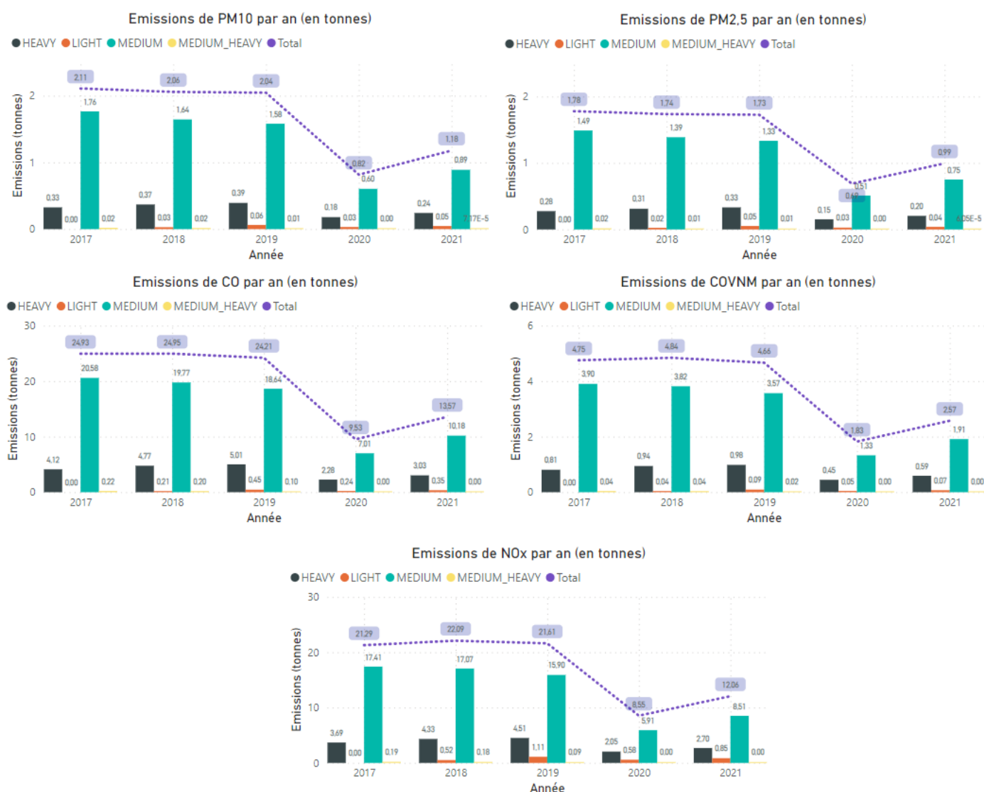
Figure 15 : Evolution pluriannuelle des émissions en tonnes de NO x , HC, CO et PM 10 avec les facteurs CDG 2018 pour la plateforme de Paris-Orly
