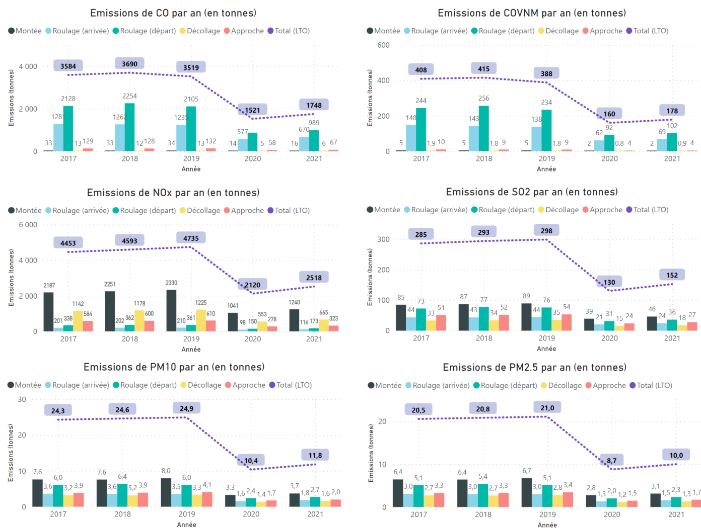
Figure 5 : Evolution des émissions par polluant (CO, COVNM, NO x , SO 2 , PM 10 , PM 2.5 ) détaillée par phase du cycle LTO à Paris-Charles de Gaulle
