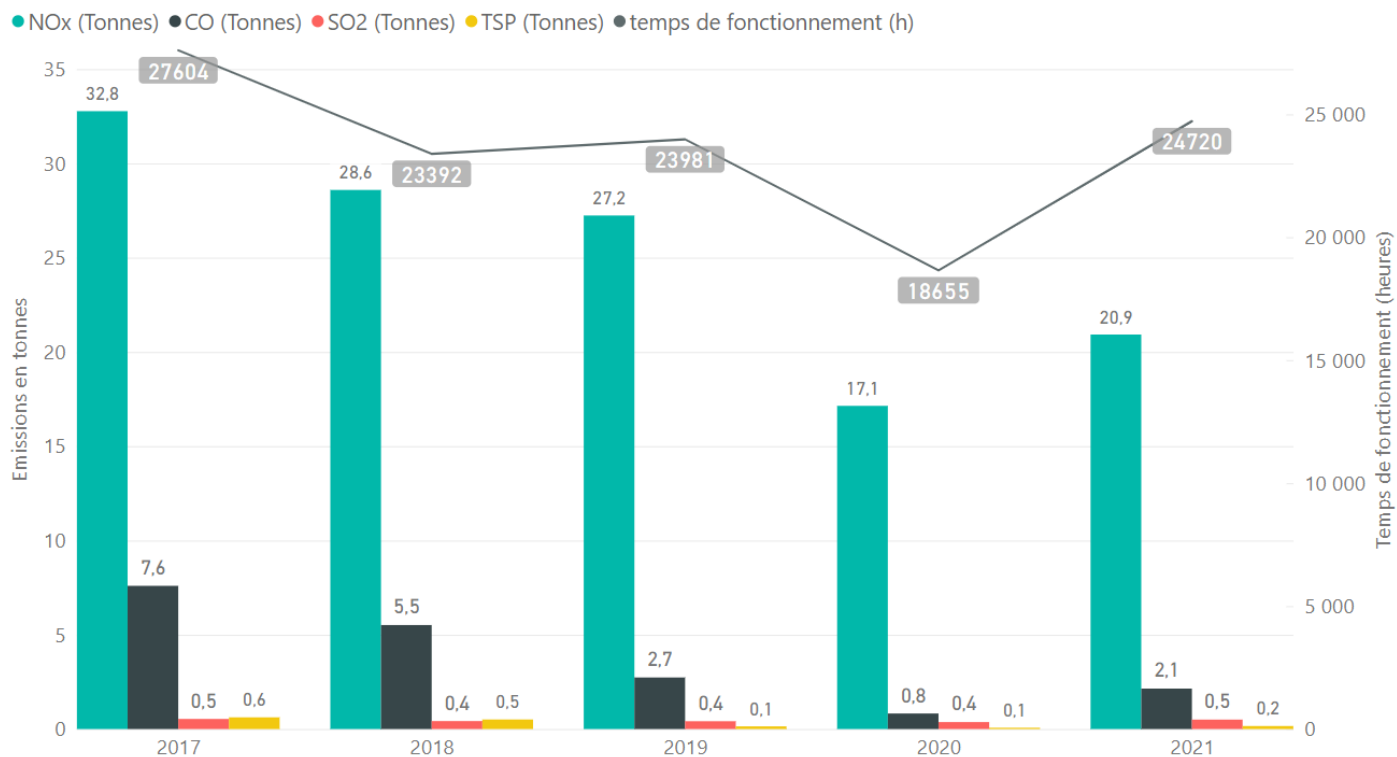
Figure 23 : Evolution pluriannuelle des émissions de NO x , CO, TSP et SO 2 et temps de fonctionnement des CTFE de Paris-Charles de Gaulle 37
