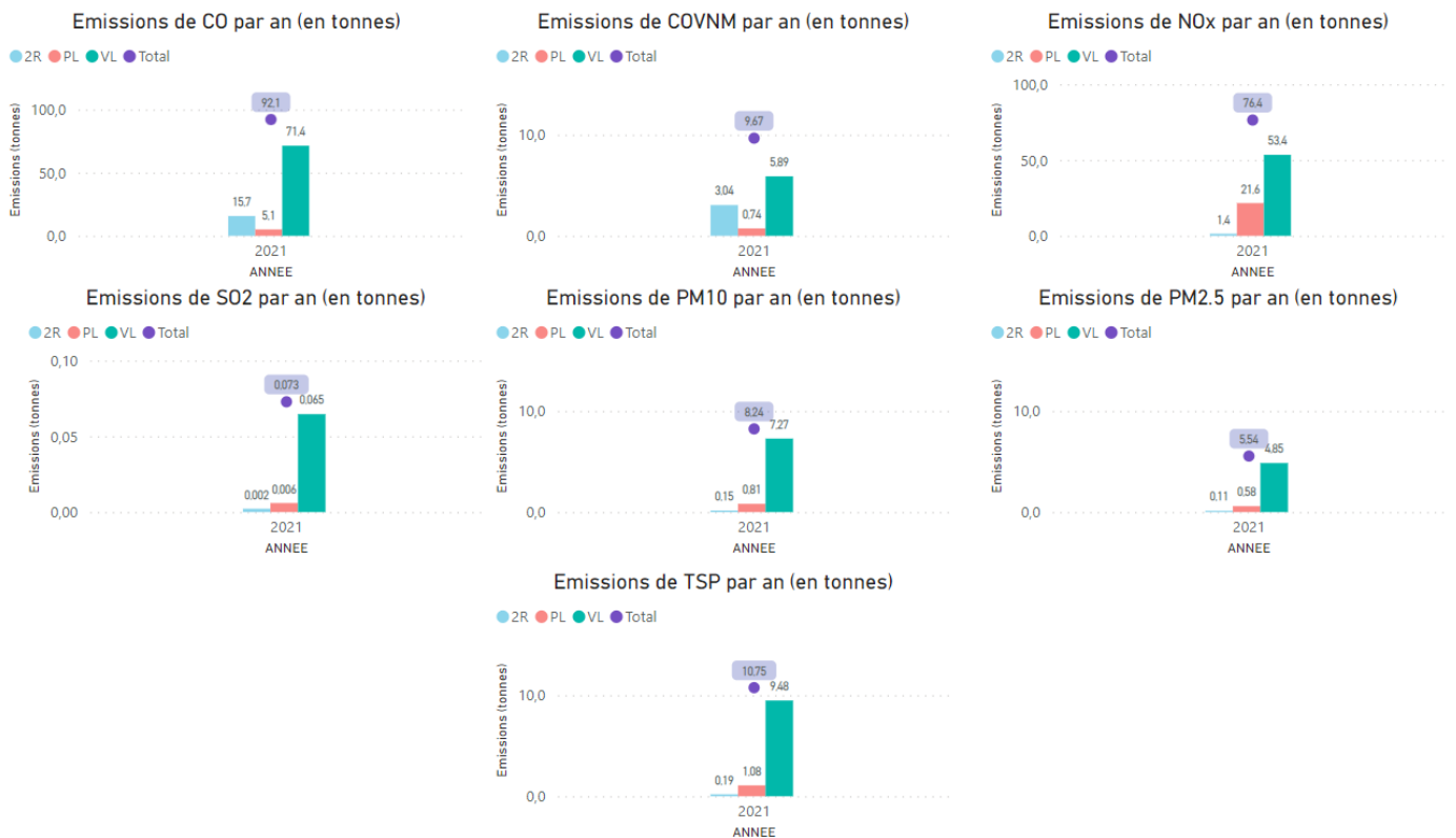
Figure 22: Emissions totales sur l'année 2021 issues du trafic routier en zone publique, par polluant et par catégorie de véhicule (2R, VL, PL) ainsi que le total des émissions sur la plateforme Paris-Orly
