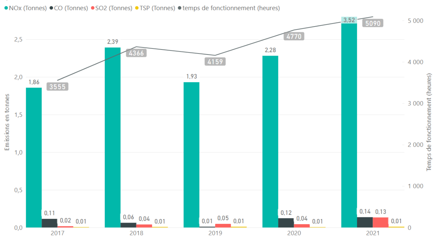
Figure 24 : Evolution pluriannuelle des émissions de NO x , CO, TSP et SO 2 et des temps de fonctionnement des CTFE de Paris-Orly
