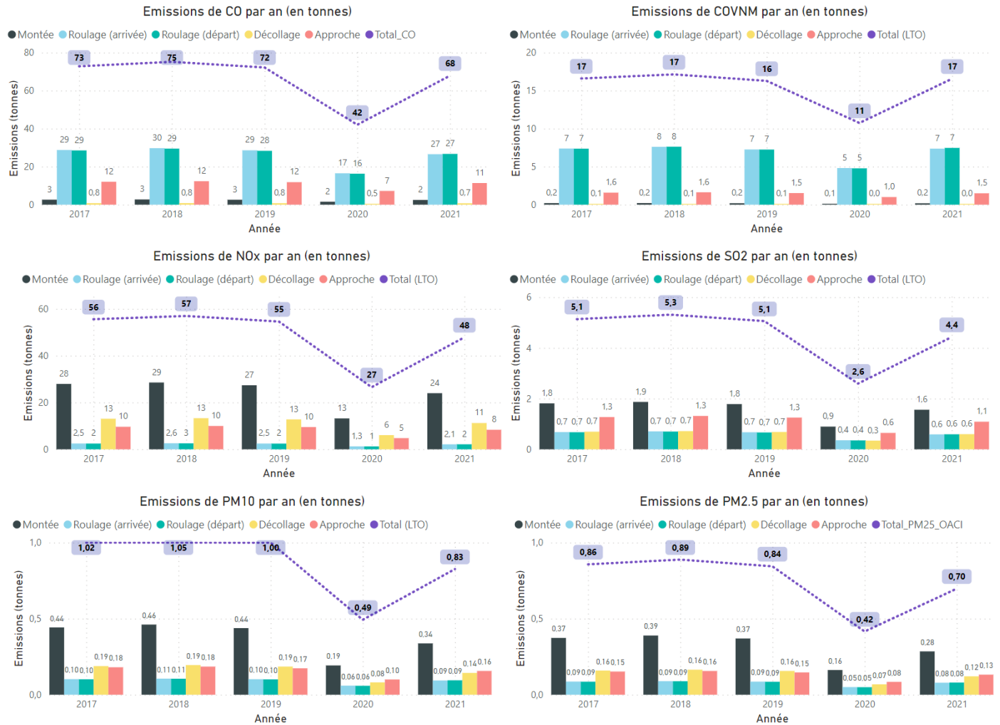
Figure 9 : Evolution des émissions par polluant (CO, COVNM, NO x , SO 2 , PM 10 , PM 2.5 ) détaillée par phase du cycle LTO à Paris-Le Bourget
