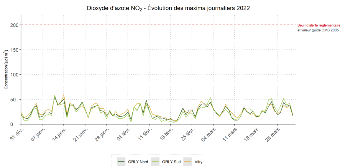
Figure 2: Dioxyde d'azote (NO 2 ) sur Paris-Orly et environs - Evolution des maximum horaires journaliers
