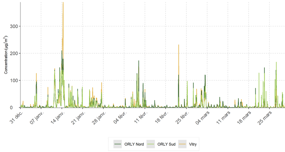
Monoxyde d'azote NO - Évolution des moyennes horaires 2022
