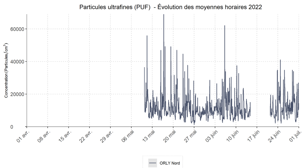
Figure 6: Particules ultrafines sur Paris-Orly - Evolution des moyennes horaires
