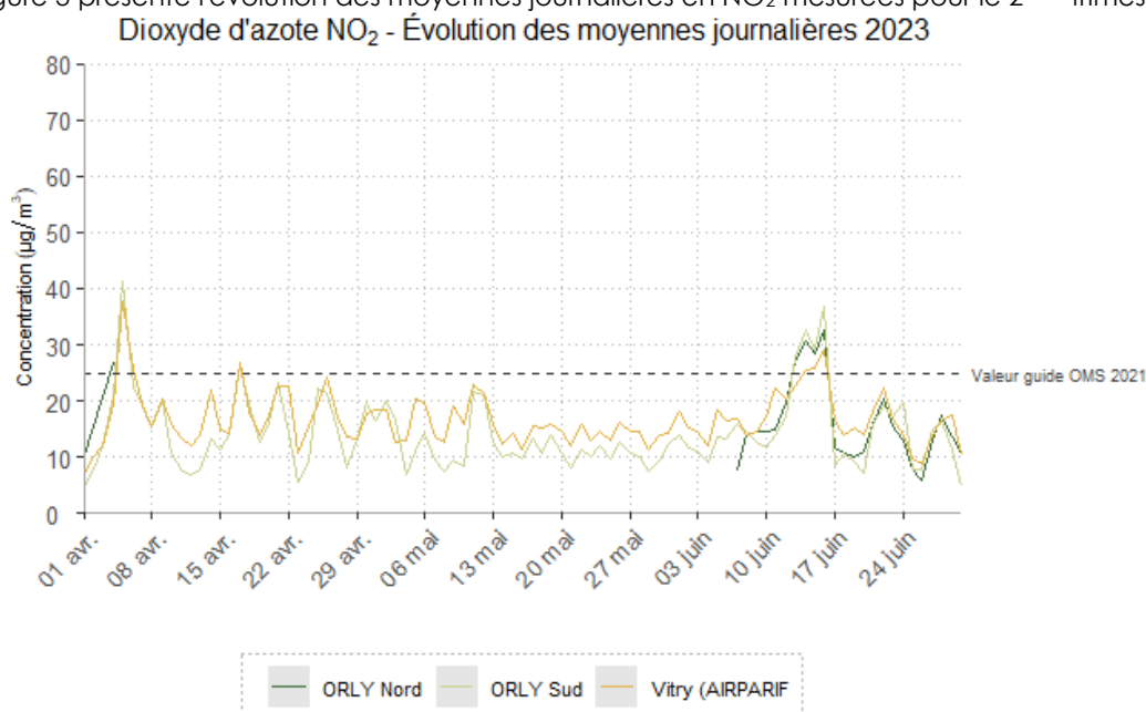
Figure 3: Dioxyde d'azote (NO 2 ) sur Paris-Orly et environs - Evolution des moyennes journalières
