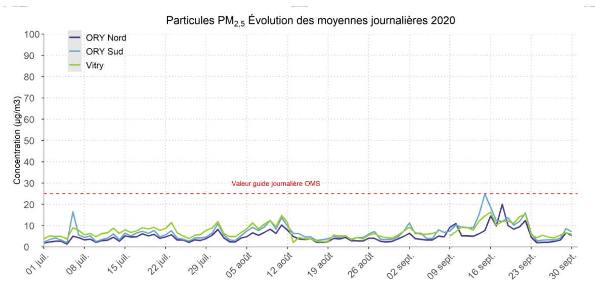
Figure 4: PM 2,5 sur Paris-Orly et environs - Evolution des moyennes journalières
