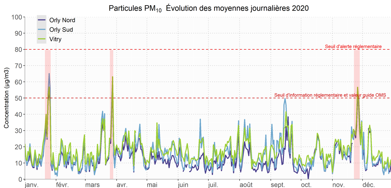
Figure 11 : Particules PM 10 sur Paris-Orly et environs
