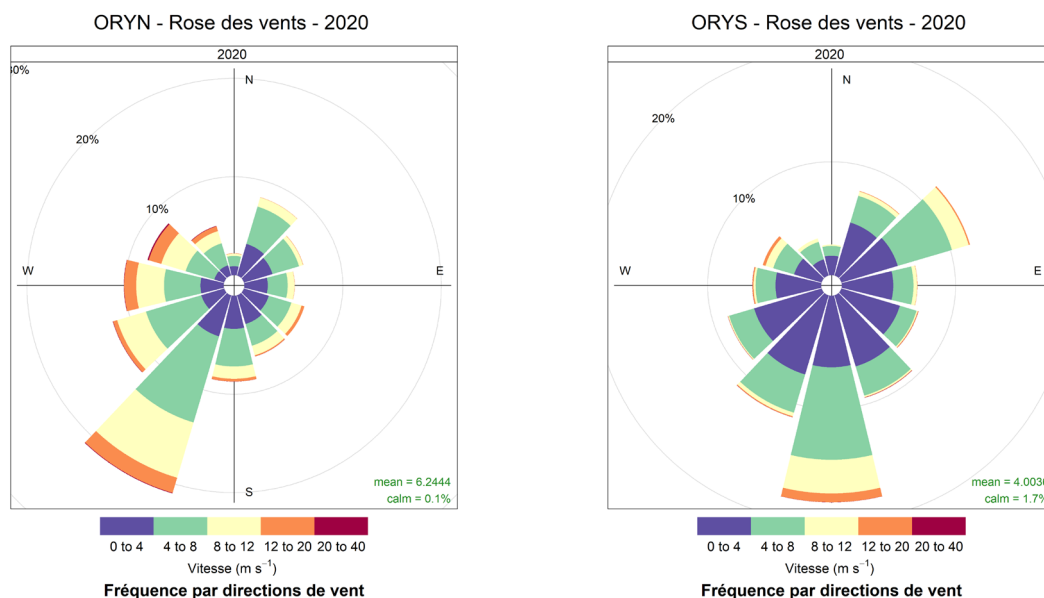
Figure 7 : Roses des vents mesurées sur les stations Orly Nord et Sud pour l'année 2020
