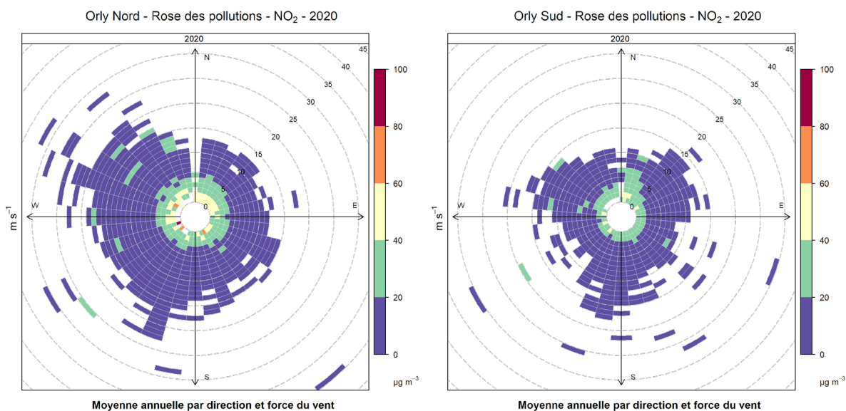
Figure 8 : Roses des pollutions des stations Orly Nord et Sud en NO 2 pour l'année 2020
