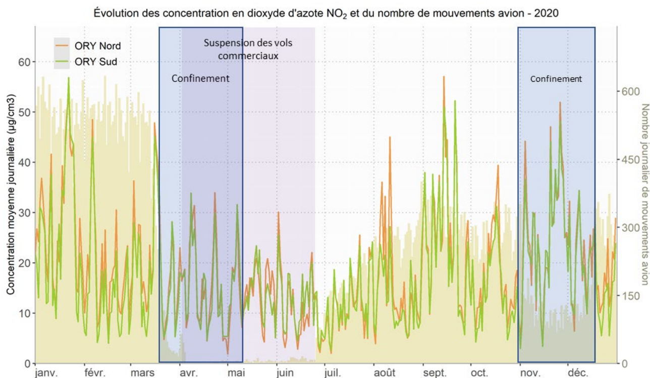
Figure 10: Evolution des concentrations moyennes journalières en NO 2 et du nombre de mouvements avion pour l'année 2020
