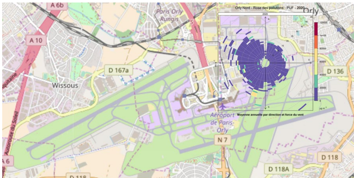
Figure 25 : Roses des pollutions des particules ultrafines sur la station Orly Nord pour l'année 2020
