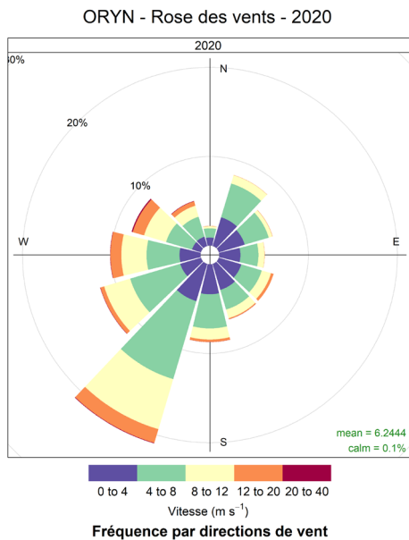
Figure 23 : Roses des vents mesurées sur la station Orly Nord pour l'année 2020
