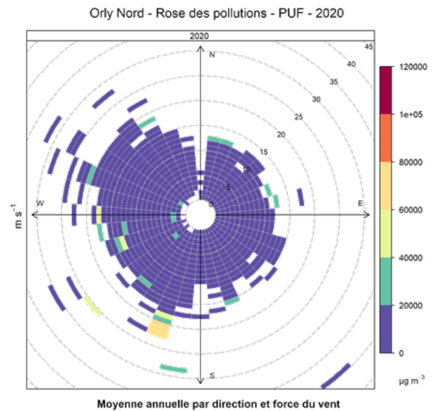
Figure 24 : Roses des pollutions des particules ultrafines sur la station Orly Nord pour l'année 2020
