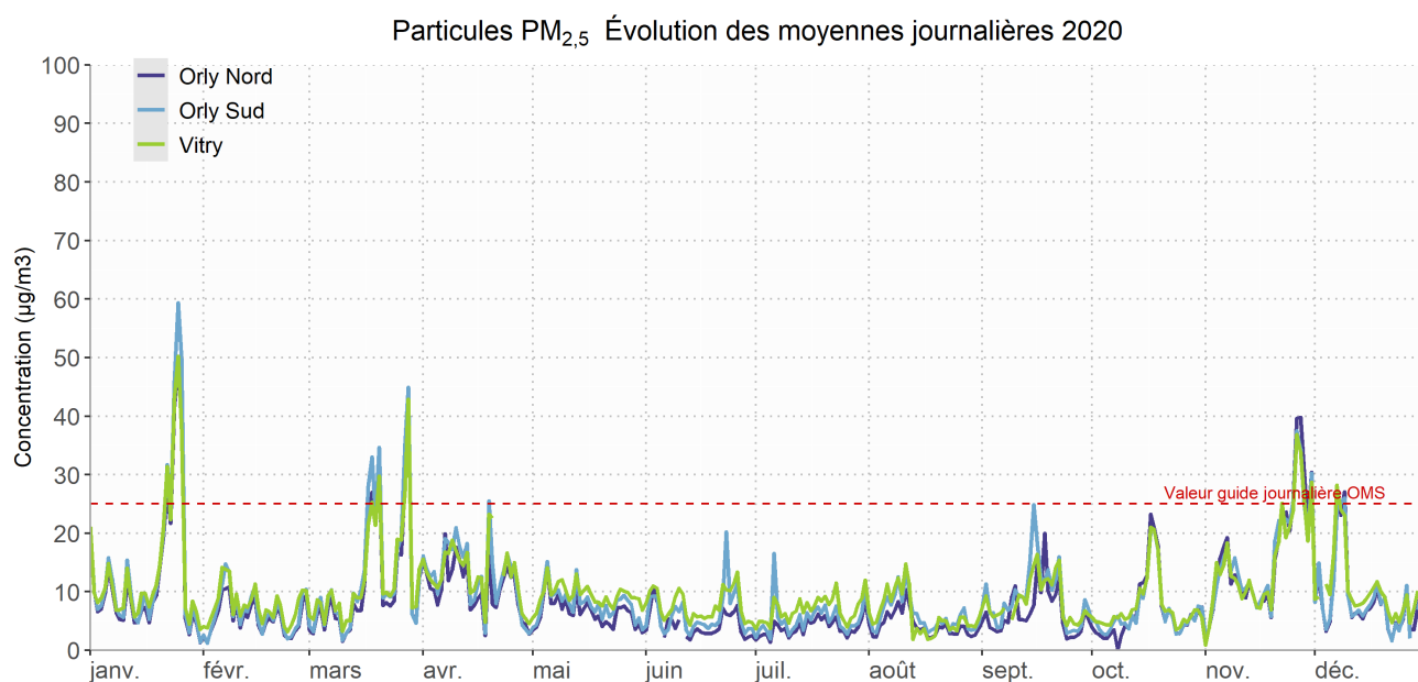
Figure 12 : Particules PM 2,5 sur Paris-Orly et environs
