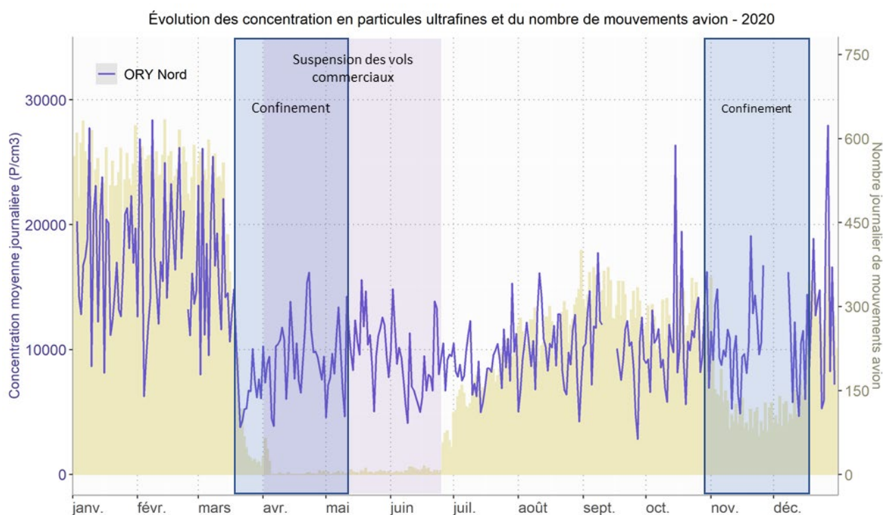
Figure 26: Particules ultrafines à la station Nord de Paris - Orly et nombre de mouvements avion
