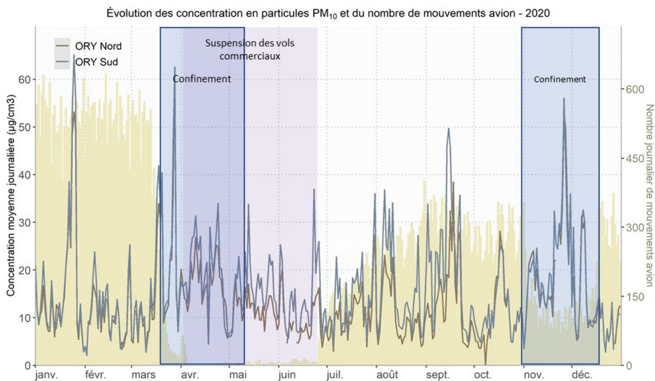
Figure 19: Evolution des concentrations moyennes journalières en PM 10 et du nombre de mouvements avion pour l'année 2020
