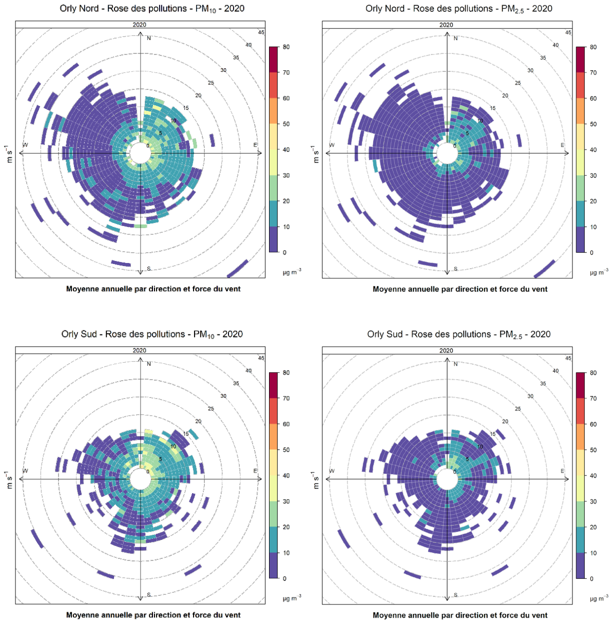
Figure 17 : Roses des pollutions des stations Orly Nord et Orly Sud en PM 10 et PM 2,5 pour l'année 2020.
