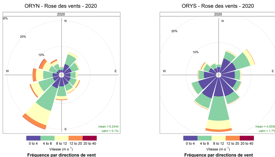
Figure 16 : Roses des vents mesurées sur les stations Orly Nord et Sud pour l'année 2020
