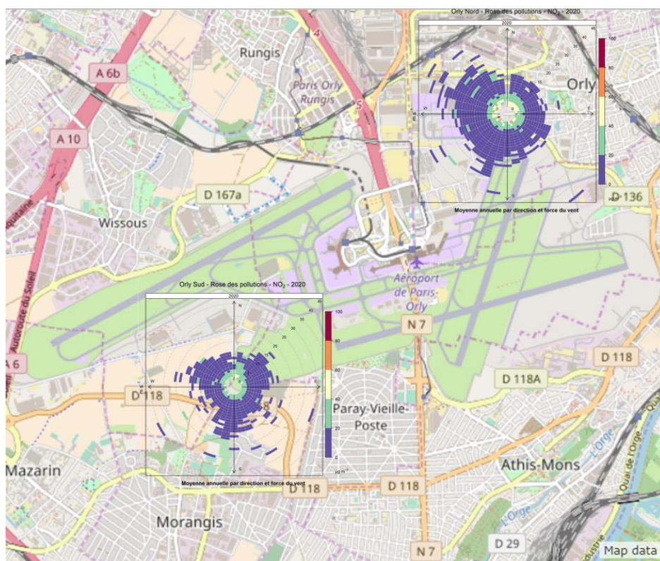
Figure 9 : Roses des pollutions NO 2 à Paris-Orly
