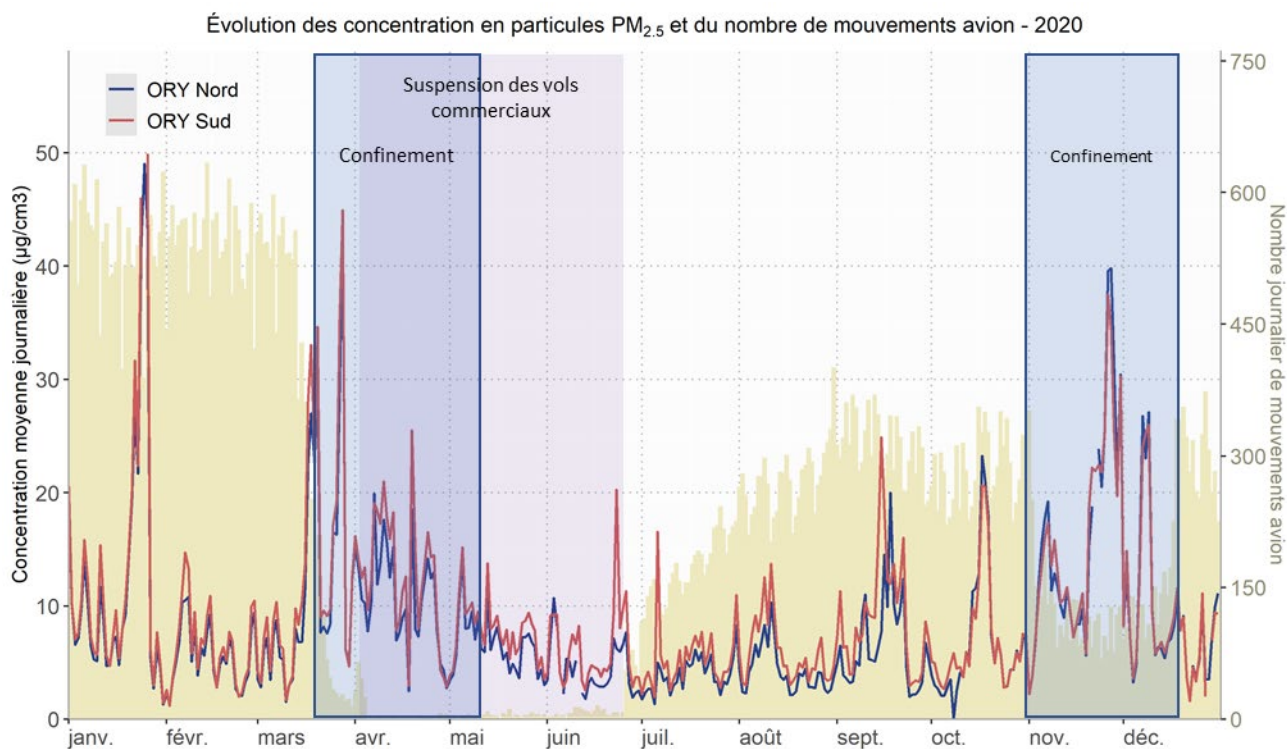
Figure 20: Evolution des concentrations moyennes journalières en PM 2,5 et du nombre de mouvements avion pour l'année 2020
