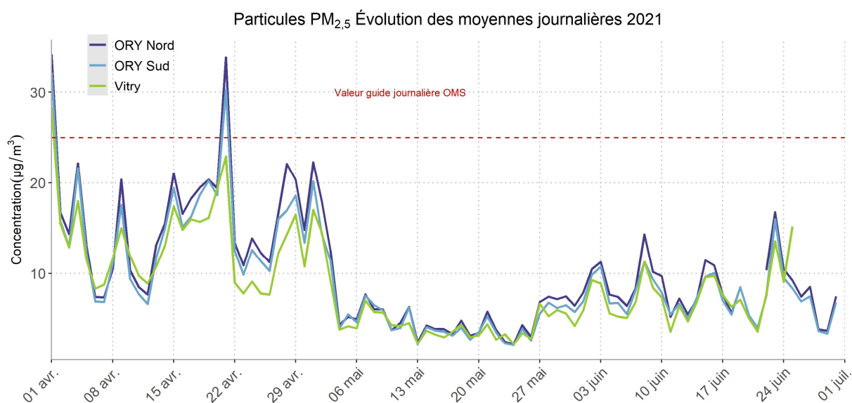
Figure 4: PM 2,5 sur Paris-Orly et environs - Evolution des moyennes journalières
